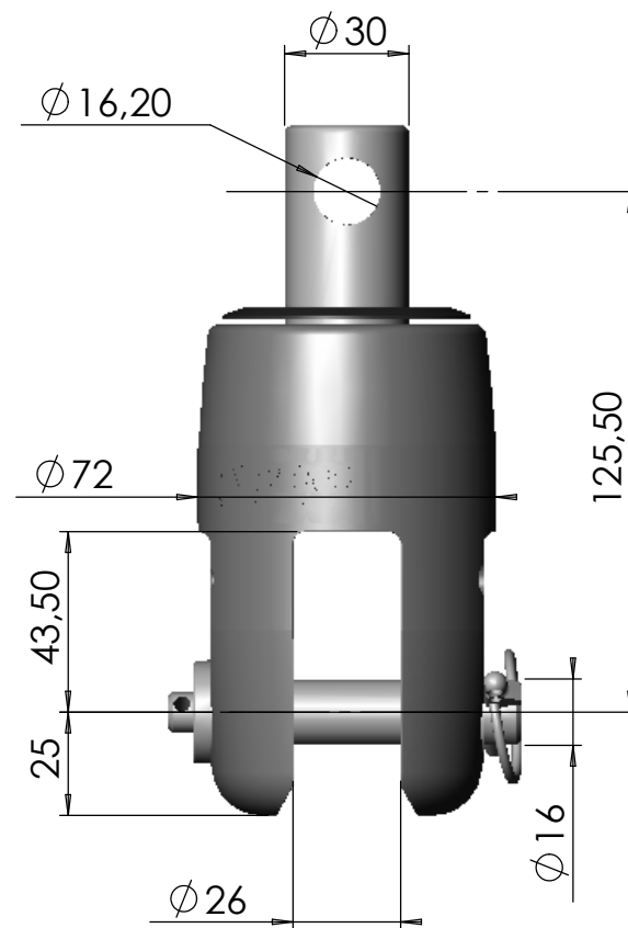
Manille Ø16HR / Ø16HR Shackle Poids/weight : 518g
