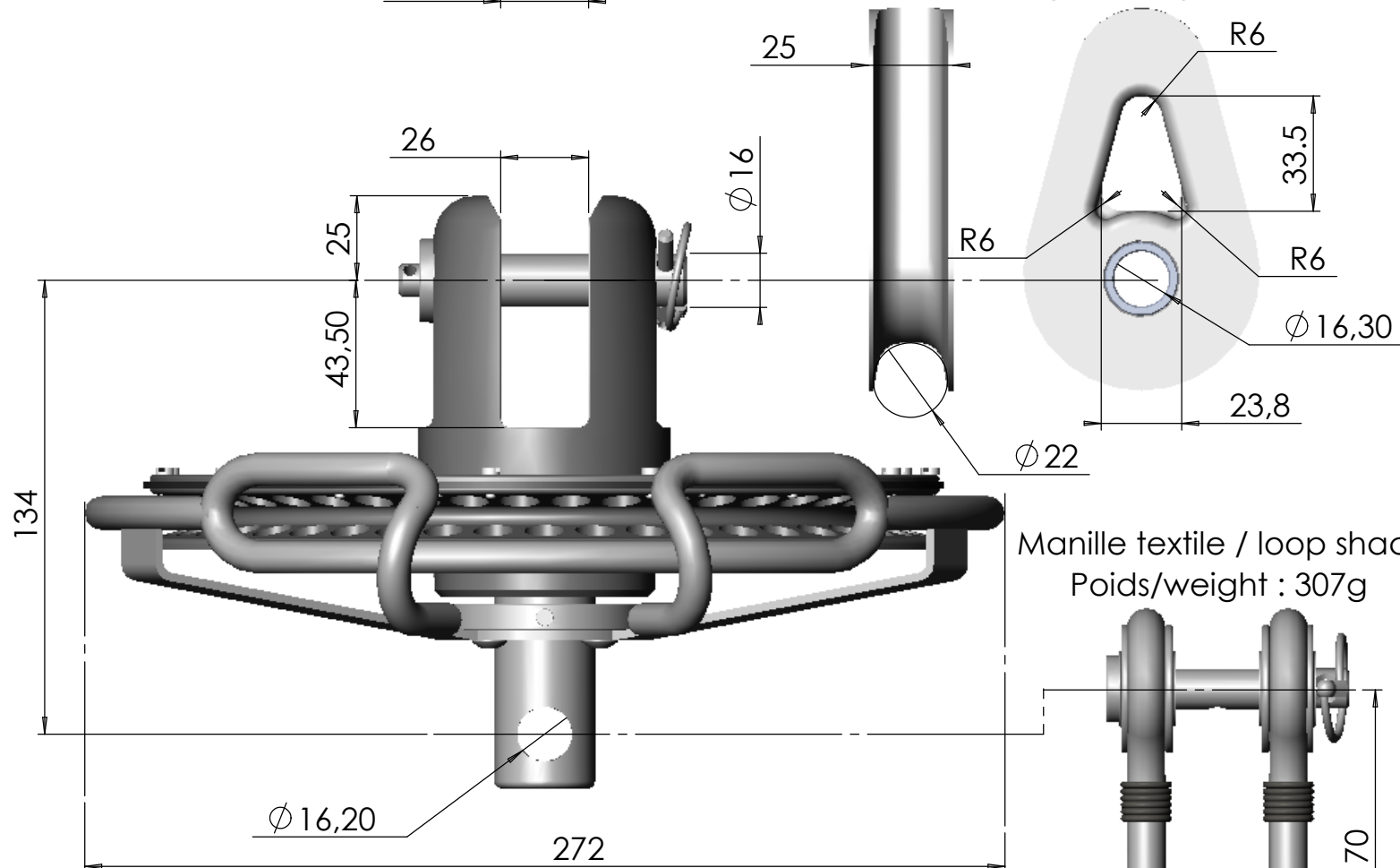
Cosse / thimble Poids/weight : 187g
